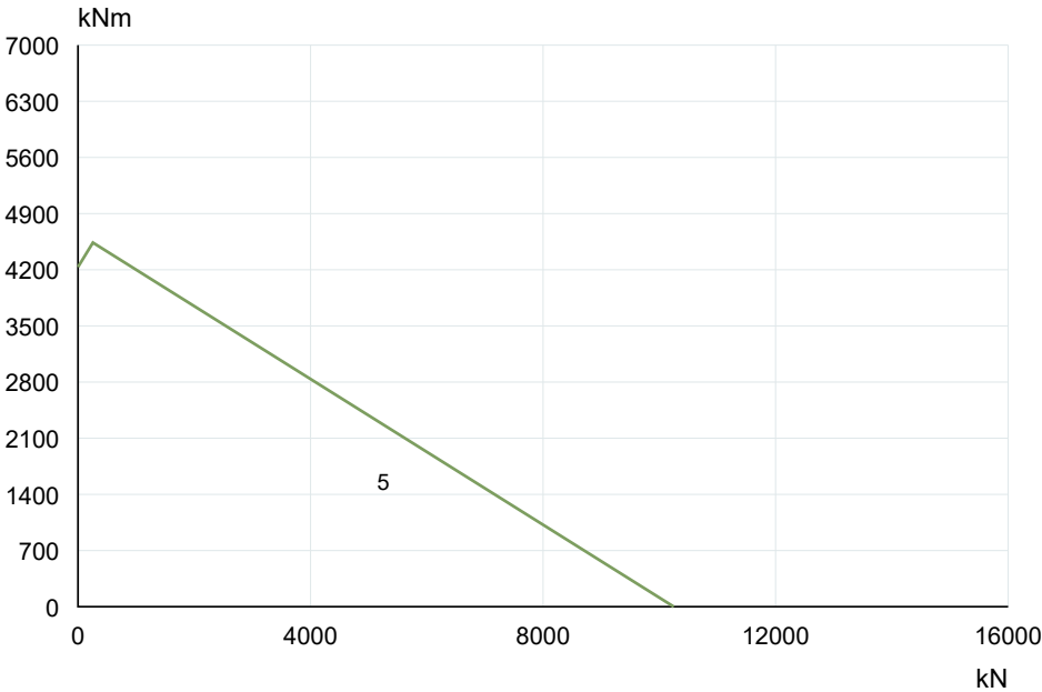
VS218A00 · Curva originale 1S 5 · PDF p24
