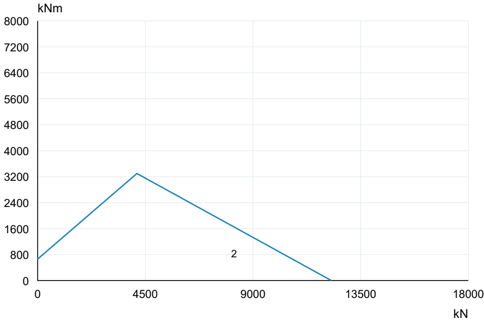
VS165B00 · Curva originale 2S 2 · PDF p15
