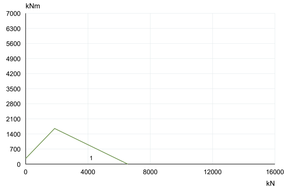
VS153A00 · Curva original 1S 1 · PDF p24
