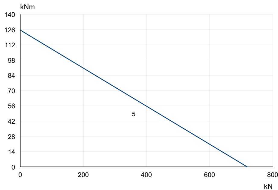
VS100UE00 · Curva originale U 5 · PDF p6
