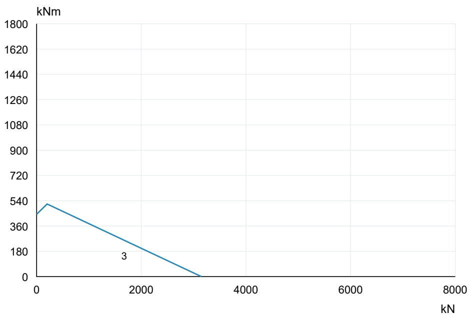
VS098B02 · Curva original 2S 3 · PDF p11
