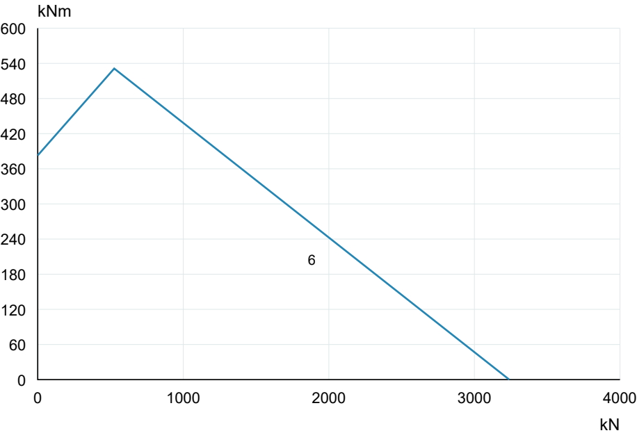
VS077B00 · Curva originale 2S 6 · PDF p7
