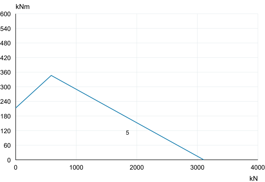
VS069B00 · Curva originale 2S 5 · PDF p7
