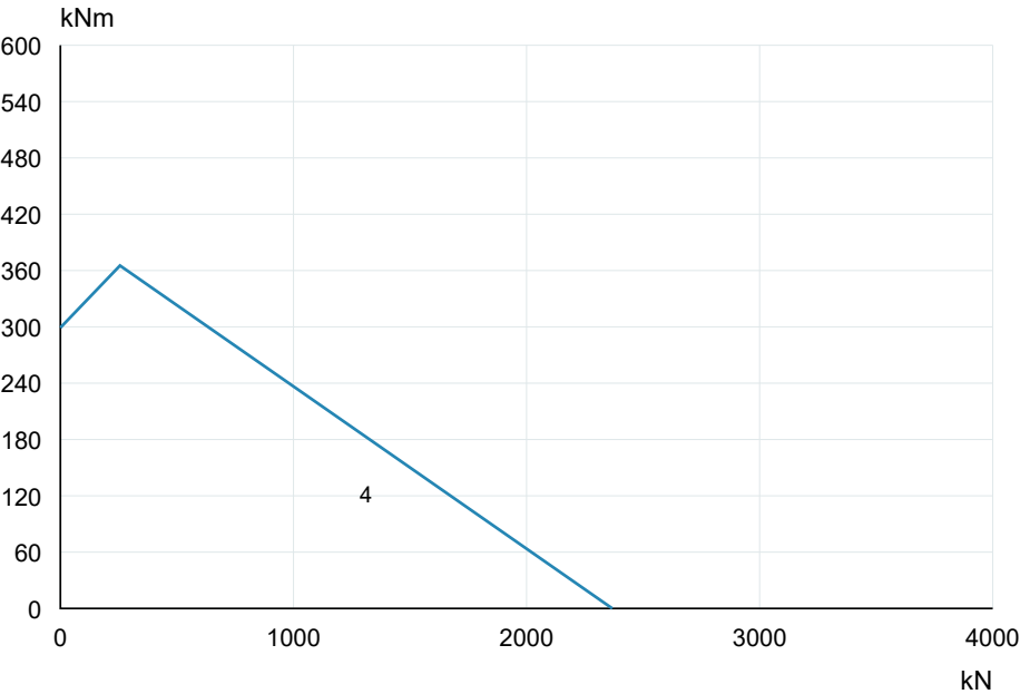
VS068B00 · Curva originale 2S 4 · PDF p7
