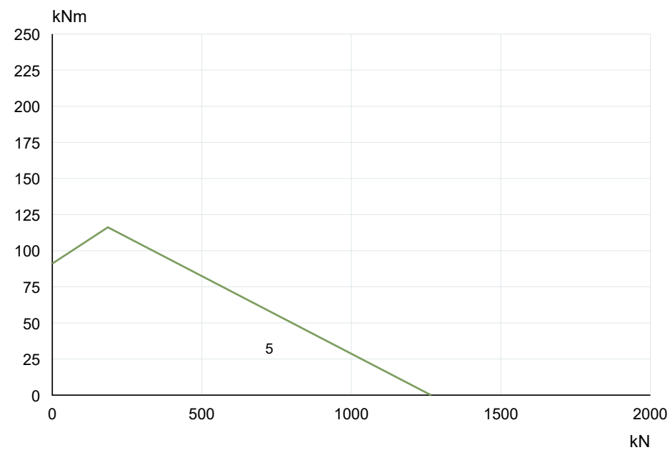
VS064A08 · Curva original 1S 5 · PDF p20
