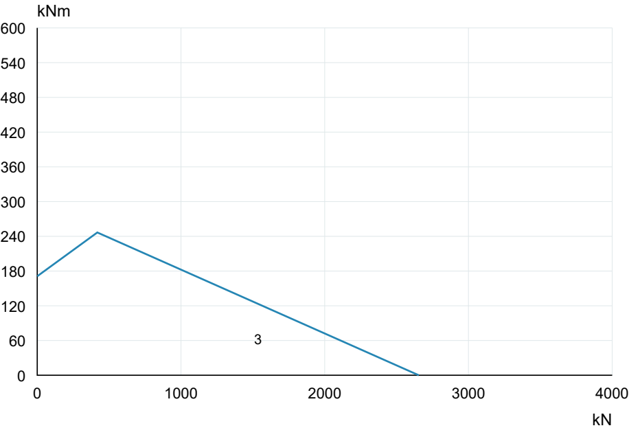
VS057B01 · Curva originale 2S 3 · PDF p7
