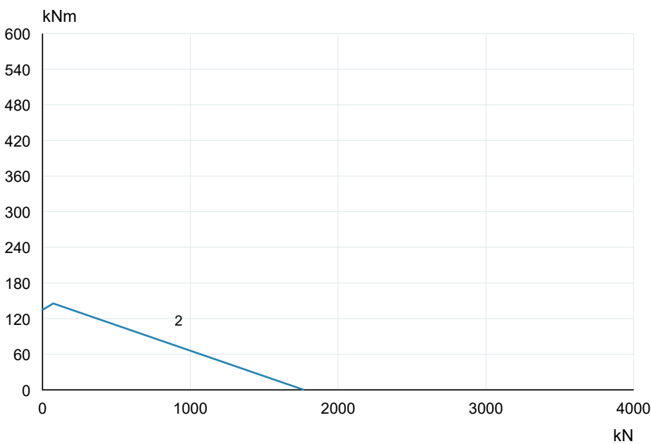
VS052B00 · Исходная кривая 2S 2 · PDF стр. 7
