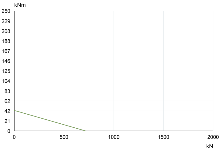
La Leonessa VS040A00 — Curva de capacidade de carga
