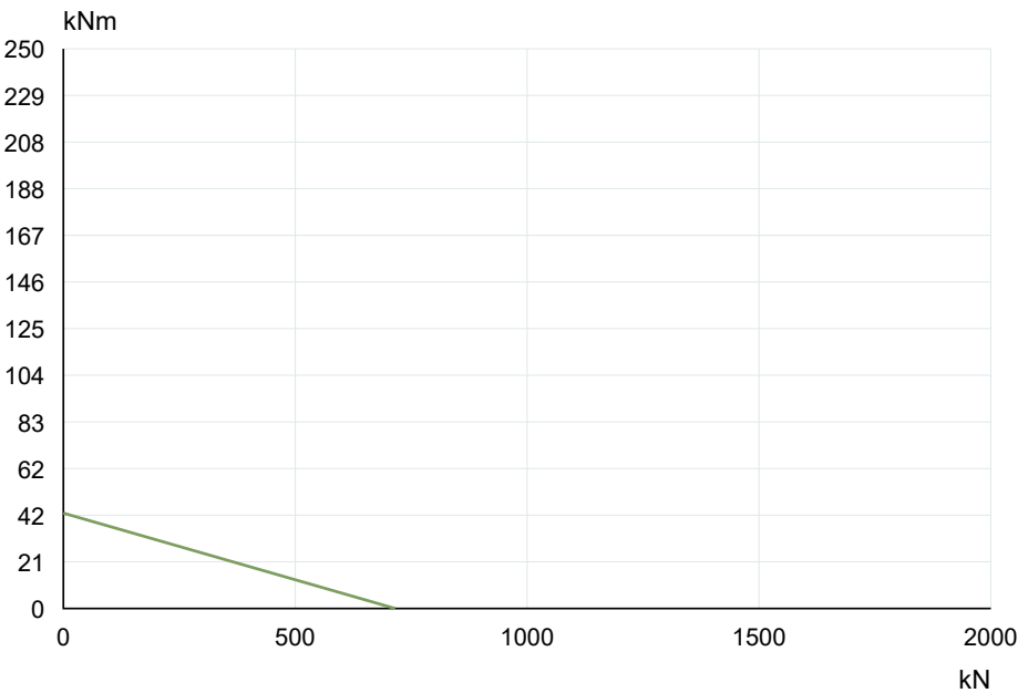
La Leonessa VS040A00 — Curva di capacità di carico
