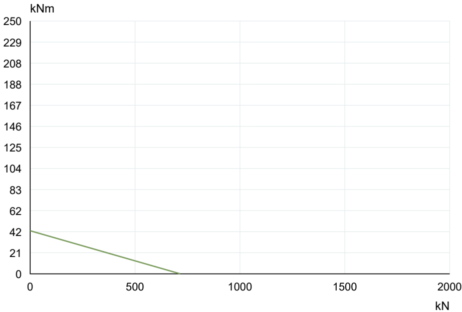
La Leonessa VS040A00 — Tragfähigkeitskurve
