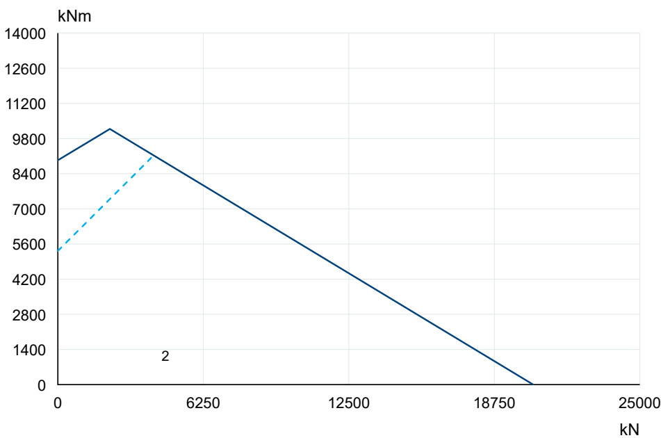
VR255E00 · Curva originale VRE-32 2 · PDF p7
