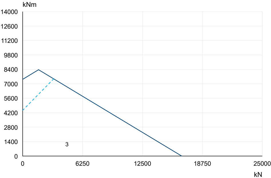
VR242I00 · Curva originale VRI-25 3 · PDF p10
