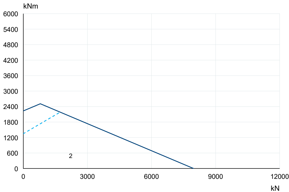
VR154I00 · Curva originale VRI-20 2 · PDF p10
