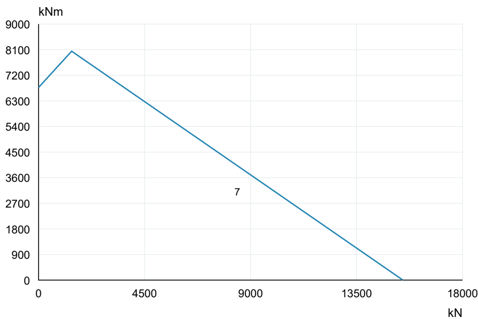
VI230B00 · Curva originale 2SI 7 · PDF p15
