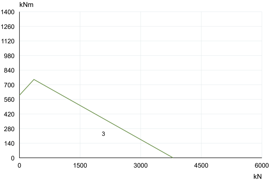
VI118A02 · Curva original 1S 3 · PDF p15
