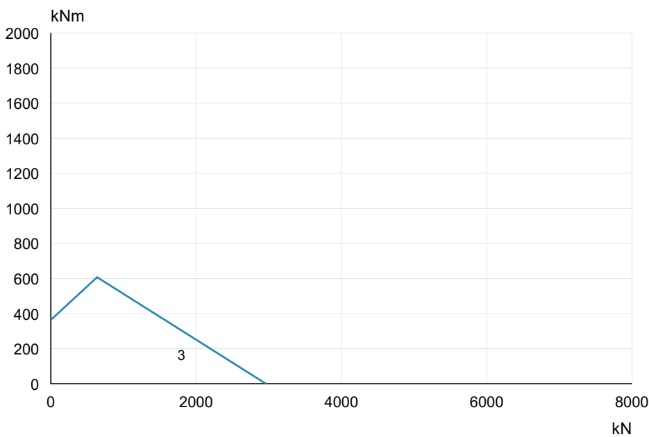
VI097B06 · Curva originale 2SI 3 · PDF p11
