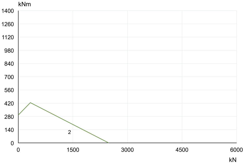
VI096A00 · Curva originale 1S 2 · PDF p15
