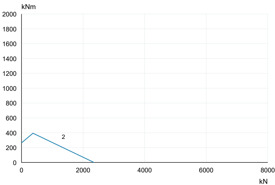
VI095B01 · Curva originale 2SI 2 · PDF p11
