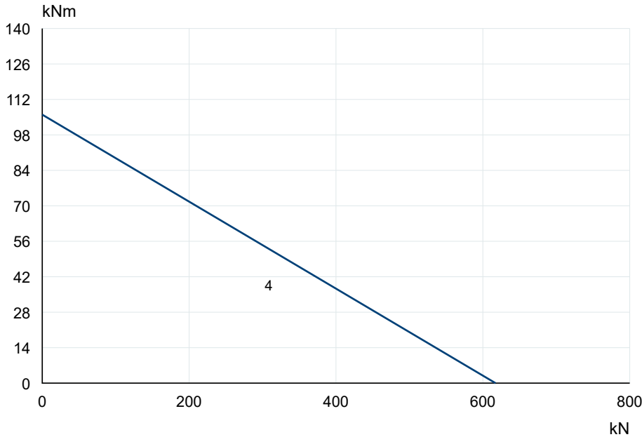
VI088UE00 · Curva originale U 4 · PDF p6
