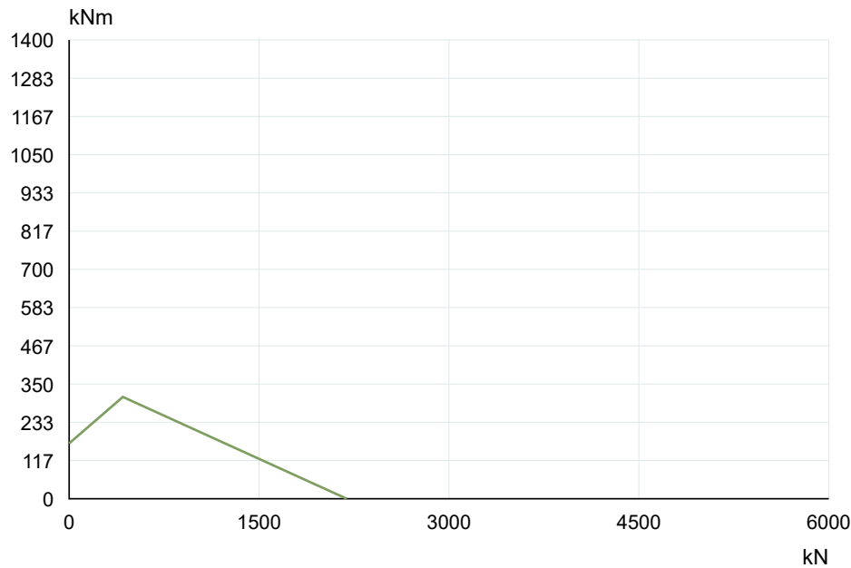
La Leonessa VI085A05 — Tragfähigkeitskurve
