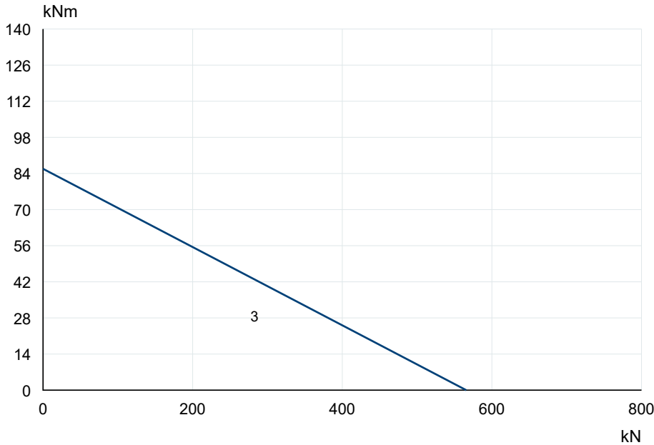
VI080UE00 · Curva originale U 3 · PDF p6
