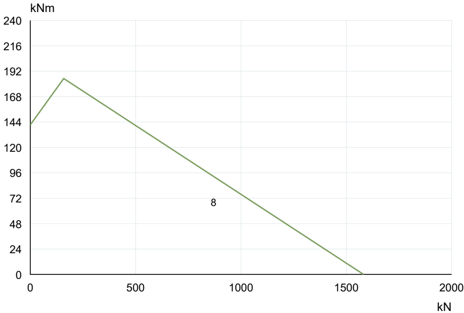
VI075A14 · Curva originale 1S 8 · PDF p13
