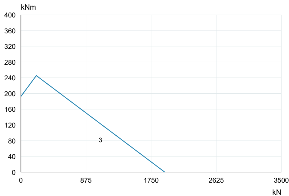
VI070B00 · Curva original 2SI 3 · PDF p7
