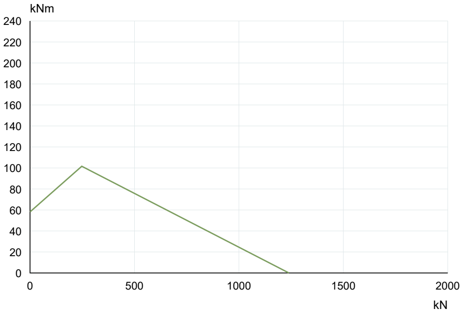
La Leonessa VI053A00 — Curva di capacità di carico
