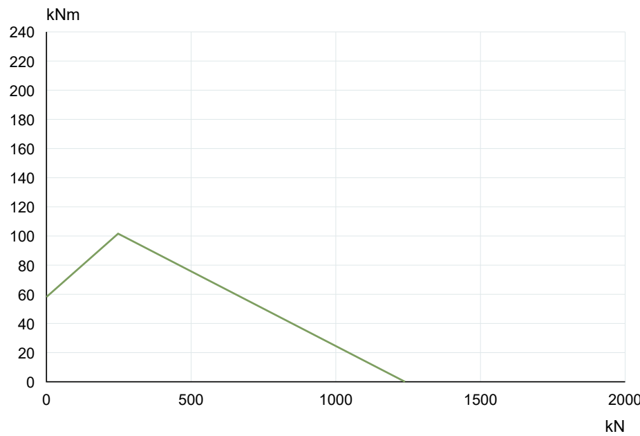
La Leonessa VI053A00 — Curva de capacidad de carga
