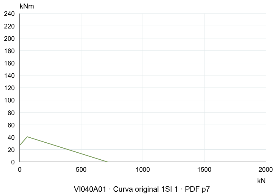
La Leonessa VI040A01 — Curva de capacidad de carga
