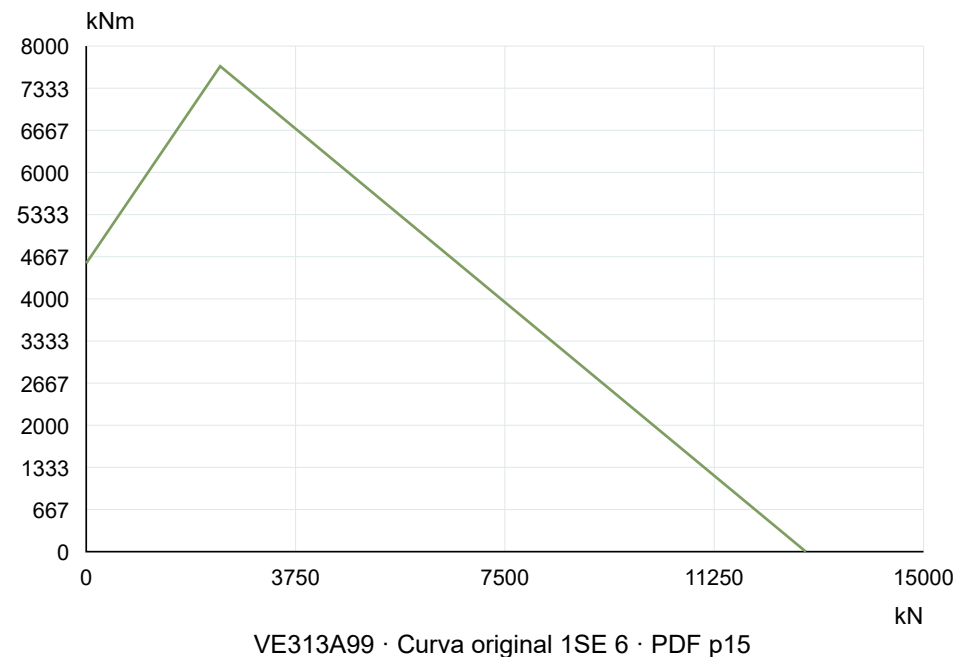
La Leonessa VE313A99 — Curva de capacidade de carga
