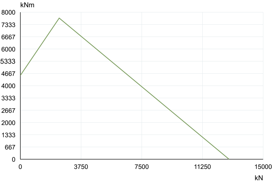
La Leonessa VE313A99 — Curva di capacità di carico
