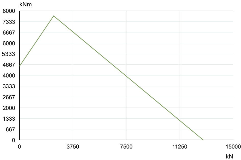
La Leonessa VE313A99 — Tragfähigkeitskurve
