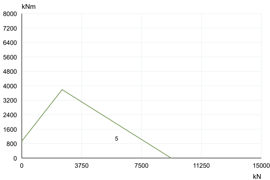
VE277A00 · Curva originale 1SE 5 · PDF p15
