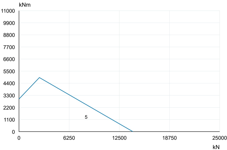
VE202B00 · Curva originale 2SE 5 · PDF p15
