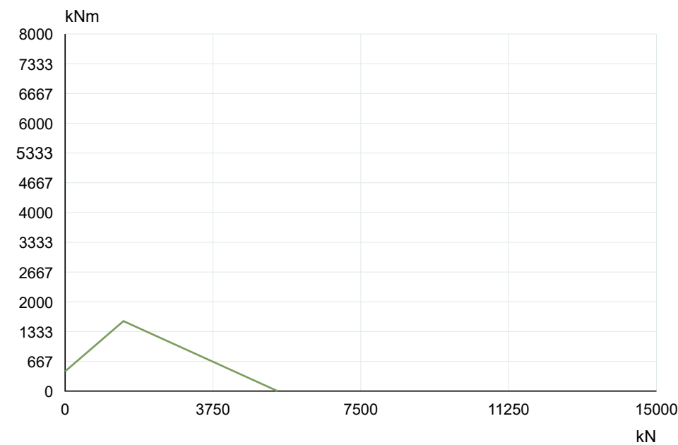
La Leonessa VE185A00 — Кривая несущей способности
