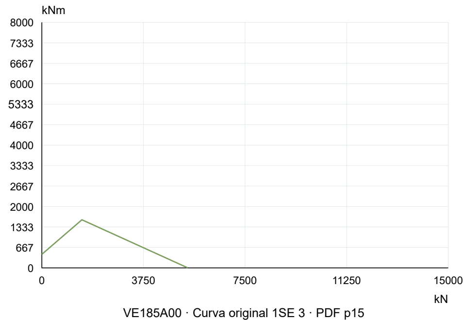
La Leonessa VE185A00 — Curva de capacidade de carga
