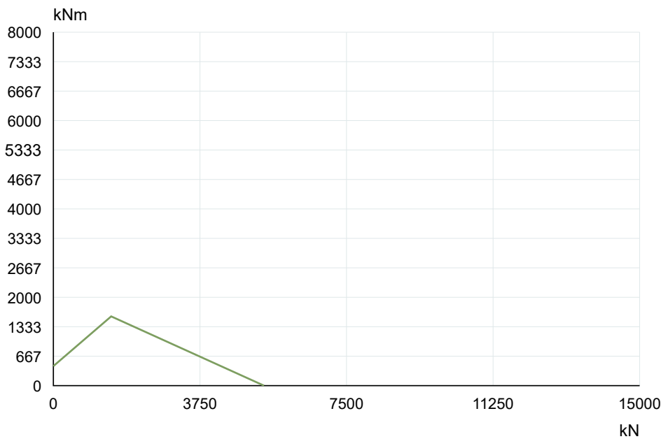
La Leonessa VE185A00 — Tragfähigkeitskurve
