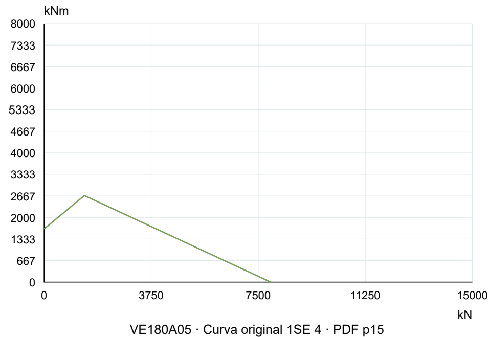
La Leonessa VE180A05 — Curva de capacidade de carga
