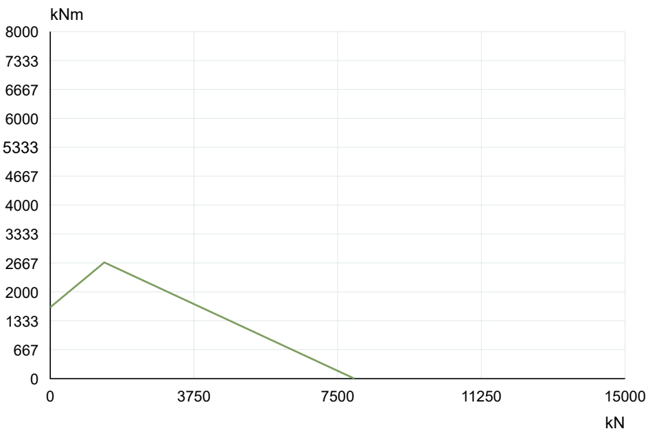
La Leonessa VE180A05 — Curva de capacidad de carga
