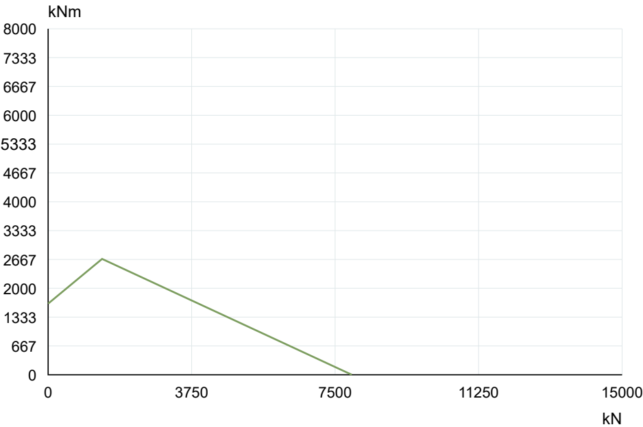
La Leonessa VE180A05 — Tragfähigkeitskurve
