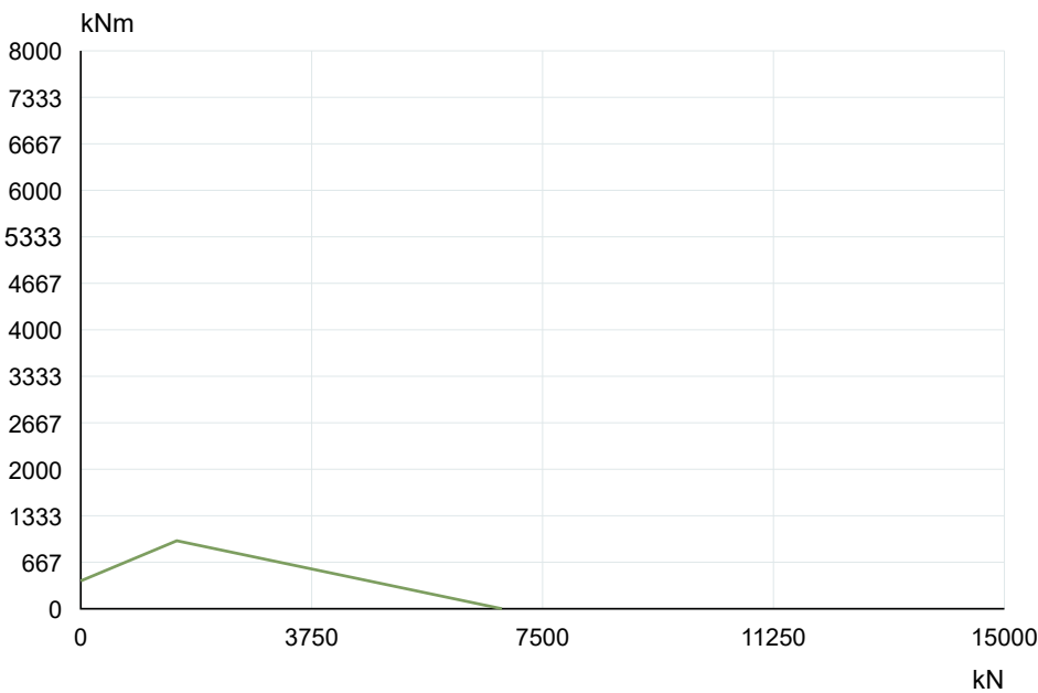
La Leonessa VE160A04 — Curva de capacidad de carga
