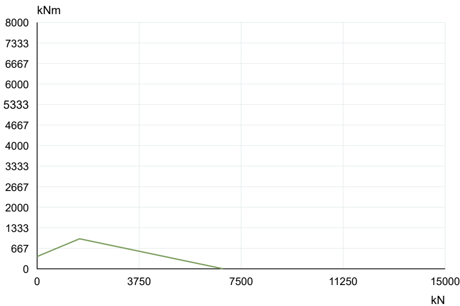
La Leonessa VE160A04 — Tragfähigkeitskurve
