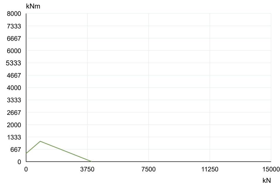
La Leonessa VE150A01 — Кривая несущей способности
