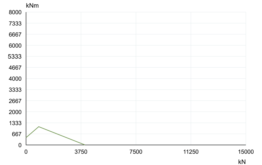
La Leonessa VE150A01 — Curva di capacità di carico
