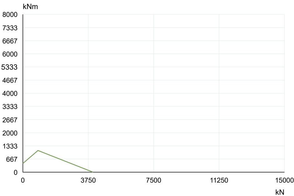
La Leonessa VE150A01 — Curva de capacidad de carga
