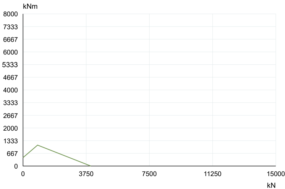
La Leonessa VE150A01 — Tragfähigkeitskurve
