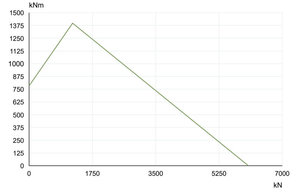
La Leonessa VE147A00 — Yük kapasitesi eğrisi
