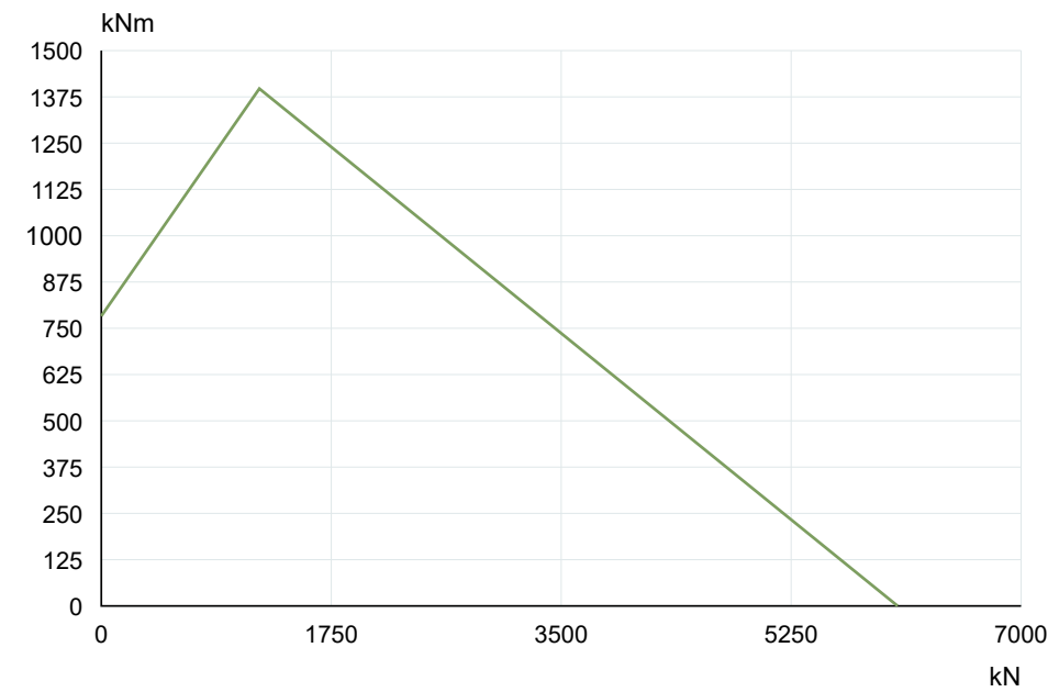
La Leonessa VE147A00 — Кривая несущей способности
