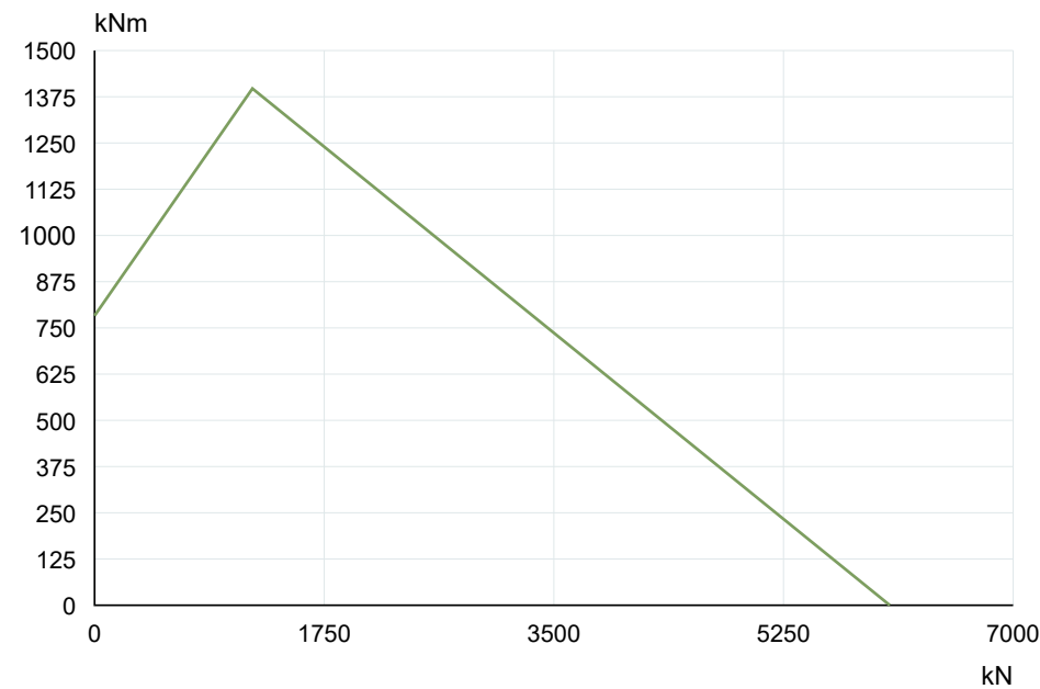
La Leonessa VE147A00 — Curva de capacidade de carga
